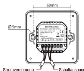
Stromversorgung Schalt Ausgang
